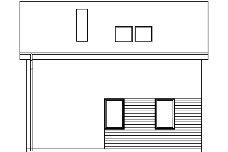
ELEWACJA ZACHODNIA
