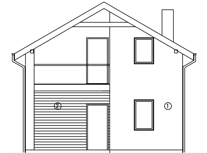
ELEWACJA PÓŁNOCNA
